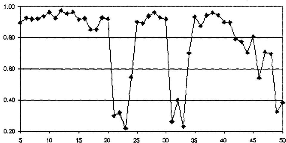
Figura 1: Ejemplo de aplicación del método de detección de inhomogeneidades relativas a partir del coeficiente de correlación.
