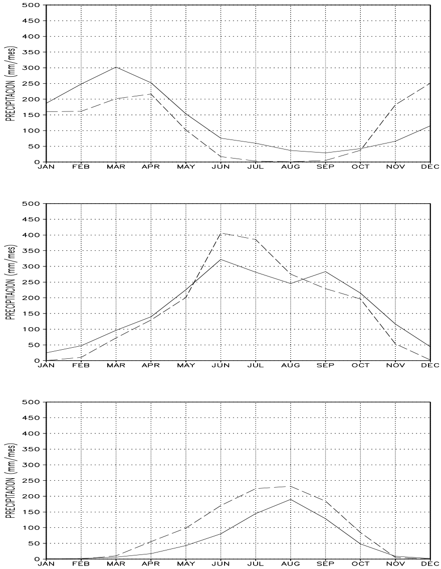
Figura 1: Climatología de la precipitación en las regiones NE (arriba), GG (medio) y SH (abajo) para las observaciones (línea continua) y la simulación con ECHAM4-ORCA (línea discontinua).
