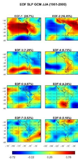
Fig. 3: EOF SLP GCM-MIROC6. Como en la figura 2, con el primer miembro del grupo r1ilplf1 para América tropical.
