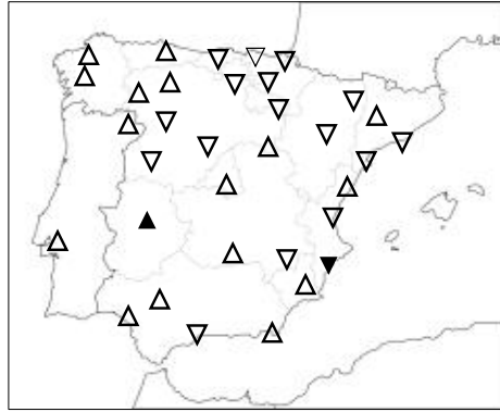
Figura 3. \Delta\bar{R}_c entre los dos subperiodos 1952-1983 y 1984-2015. Triángulo hacia arriba (abajo) indica un aumento (disminución) de la actividad convectiva en el segundo subperiodo. Triángulo lleno (vacío) indica diferencia significativa (no significativa) al nivel de confianza del 95%.
