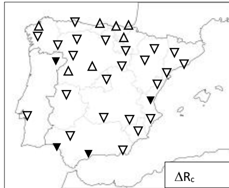
Figura 7. Variación de la actividad convectiva R_c(WeMO+) - R_c(WeMO-) durante el periodo 1952-2015. Triángulo hacia arriba (abajo) indica un aumento (disminución) durante la fase positiva de la WeMO, significativo (no significativo) al nivel de confianza del 95% si está lleno (vacío).
