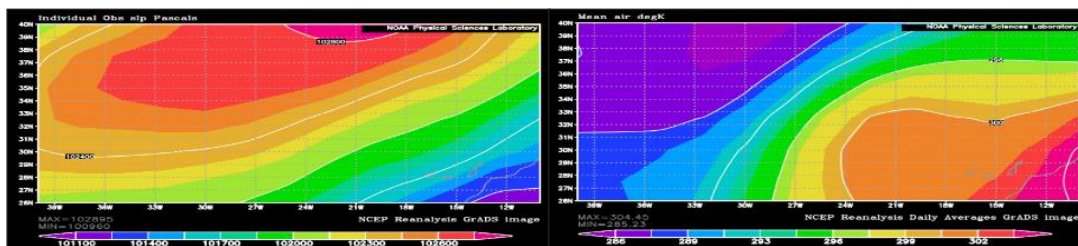
Figura 4 . A la izquierda, presión en superficie, a la derecha, temperatura a 850 hPa. Fuente: NOAA.
