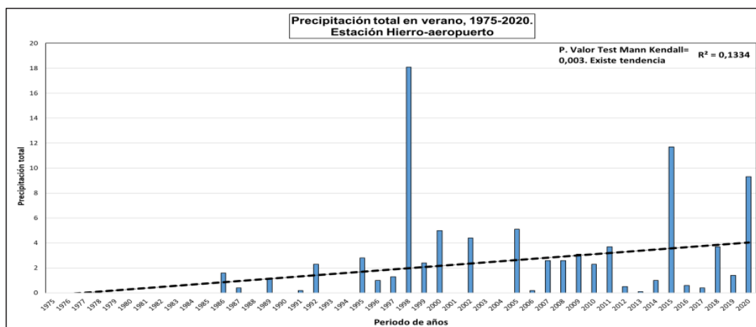
Figura 5. Precipitación total de verano, 1975 a 2020. Fuente: elaboración propia.
