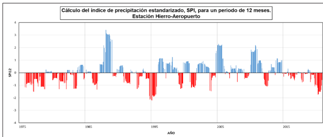
Figura 6. SPI12 calculado para la estación de El Hierro-aeropuerto. Fuente: elaboración propia.
