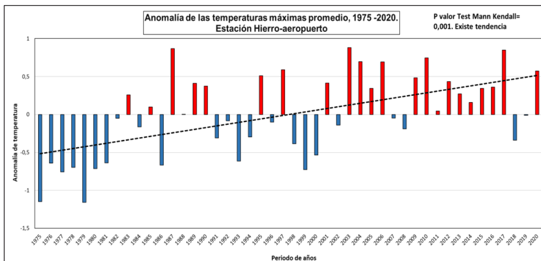
Figura 7. Anomalías de las temperaturas máximas promedio. Fuente: elaboración propia.
