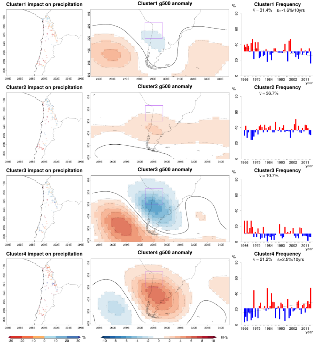
Fig. 3. Anomalías del geopotencial de 500 hPa de cada régimen, el impacto de cada uno de ellos en la precipitación de las estaciones meteorológicas y su frecuencia en el periodo 1966-2015. El marco morado indica el área empleada por el análisis cluster.
