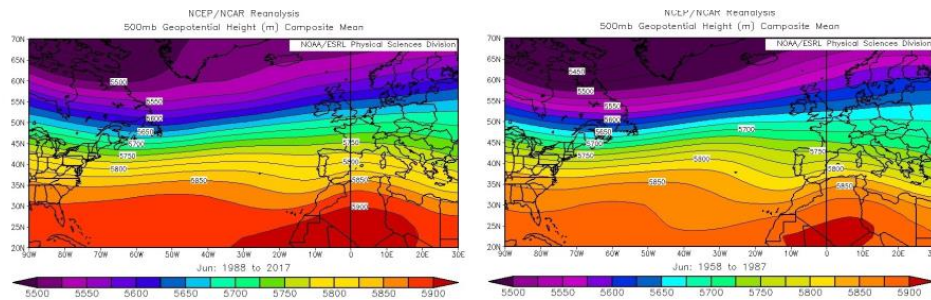
Fig. 4. Patrones medios geopotencial 500 hpa de junio en los periodos 1988-2017 (izquierda) y 1958-1987 (derecha). Fuente: Reanálisis NOAA/OAR/ESRL PSD, Boulder, Colorado, USA, de su página web en http://www.esrl.noaa.gov/psd/
