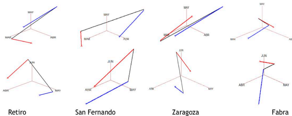
Fig. 9. Diagramas triangulares mostrando la evolución secular de la distribución de la precipitación a lo largo de los meses de marzo, abril y mayo (arriba) y abril, mayo, junio (abajo), en cuatro observatorios con series largas representativos de diversas regiones peninsulares para las veintenas 1937-1957, 1958-1977, 1978-1997 y 1998-2017. Se han utilizado los mismos criterios que en la figura 8 para la representación.
