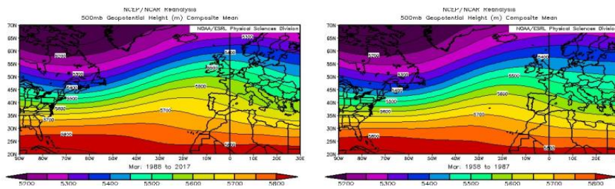
Fig. 7. Patrones medios geopotencial 500 hpa de marzo en los periodos 1988-2017 (izquierda) y 1958-1987 (derecha). Fuente: Reanálisis NOAA/OAR/ESRL PSD, Boulder, Colorado, USA, de su página web en http://www.esrl.noaa.gov/psd/
