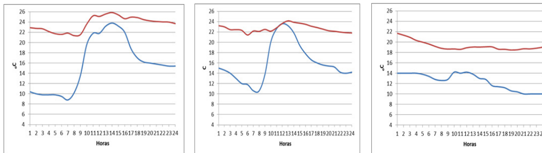
Figura 2. Marcha diaria de la temperatura (°C) en la costa (roja, LV) y a media montaña (azul, Xalapa), a) dos días antes de la llegada del frente frío (izquierda, 5/dic/2011), b) un día antes (centro, 6/dic/2011), y c) durante el frente (derecha, 7/dic/2011).
