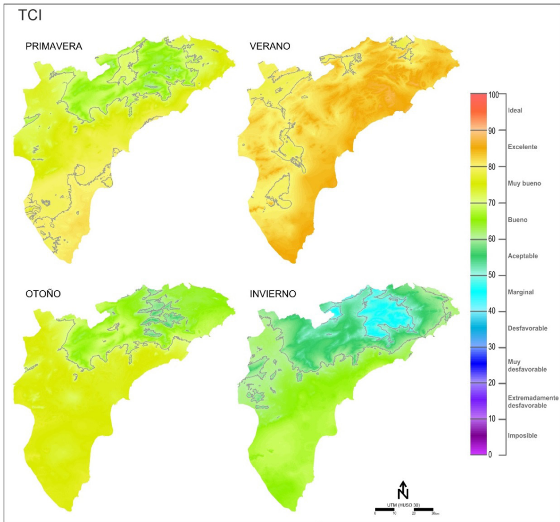
Figura 1. TCI de referencia (actual) calculado para cada estación del año.
