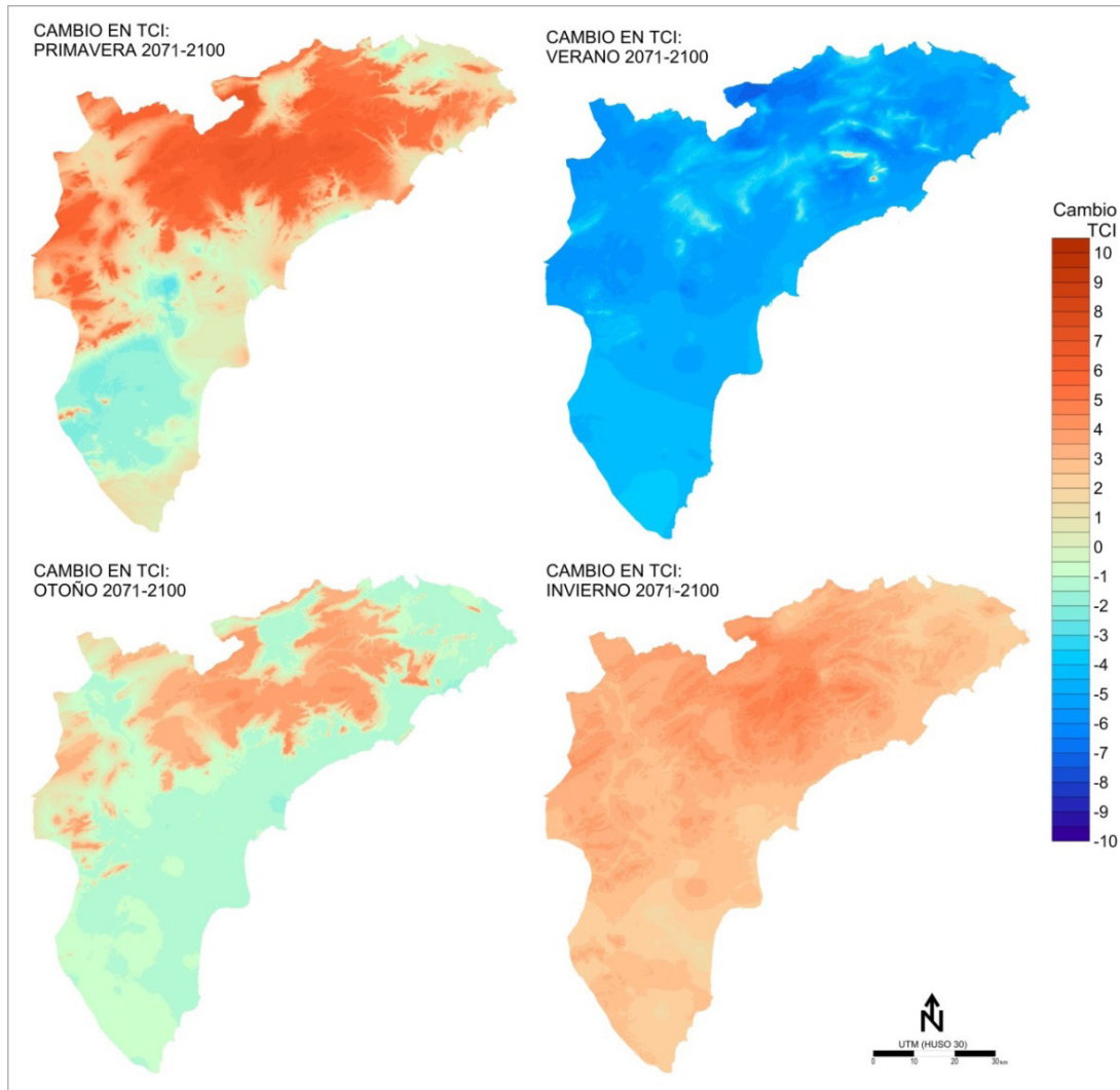
Figura 2. Cambio previsto en unidades del TCI para el periodo 2071-2100 con respecto al TCI de referencia, según la proyección climática utilizada en el estudio.
