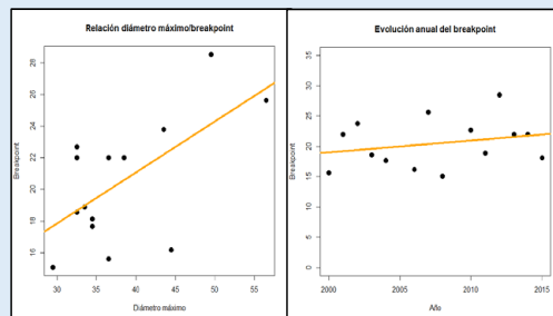
Fig. 3. Izquierda: relación entre el diámetro máximo de granizo en un año y el breakpoint en su distribución. Derecha: Evolución anual y tendencia del breakpoint en el periodo 2000-2015 (excluyendo 2005 y 2009).
