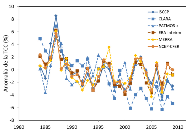
Fig. 5. Anomalías de la nubosidad total (TCC) sobre la Península Ibérica, según datos de diversos reanálisis y proyectos basados en datos de satélites. Fuente: elaboración propia, a partir de datos utilizados en Enríquez-Alonso et al. (2015).
