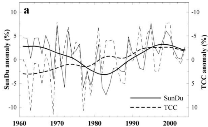
Fig. 3. Evolución de la insolación (SunDu) y de la nubosidad total (TCC) en la Península Ibérica, para el período 1961-2004. Valores anuales, expresados como anomalías relativas a la media del período 1971-2000. El eje de la nubosidad está invertido. Fuente: Sanchez-Lorenzo et al. (2009).
