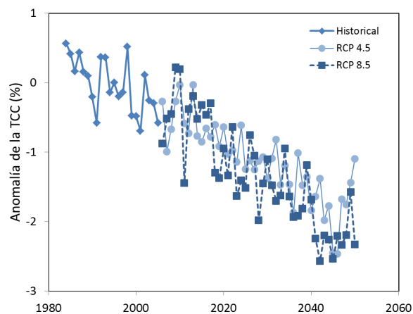
Fig. 6. Anomalías de la nubosidad total (TCC) sobre la Península Ibérica, según las simulaciones climáticas de los modelos participantes en el CMIP5.
