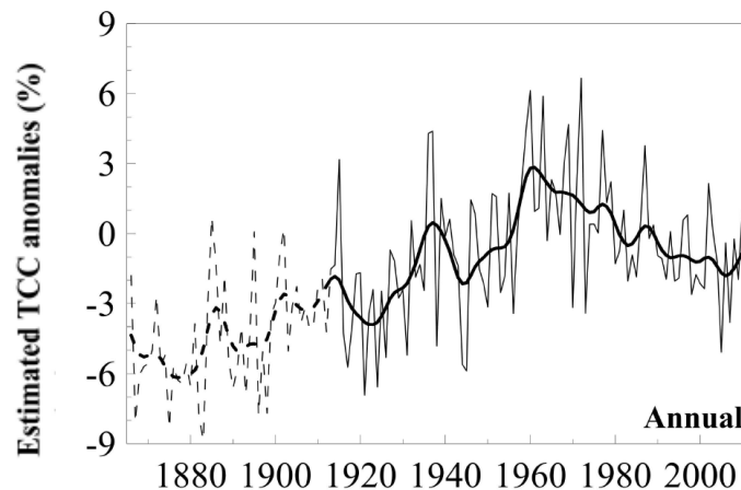
Fig. 2. Serie media de las anomalías de nubosidad total respecto a la media del periodo 1971-2000. La línea discontinua indica que antes de 1913 el número de observatorios es notablemente inferior. La línea gruesa corresponde a la curva suavizada por un filtro de pasa-bajo. Fuente: Sanchez-Lorenzo et al. (2012).
