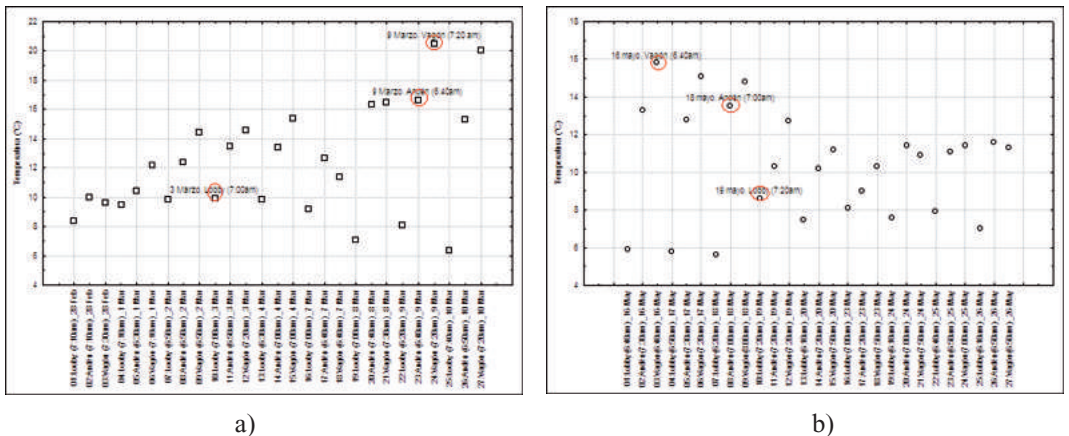
FIG. 4: Diferencia de temperatura al interior del Metro (lobby, andén y vagón) con el exterior a) en campaña fría; b) campaña cálida.
