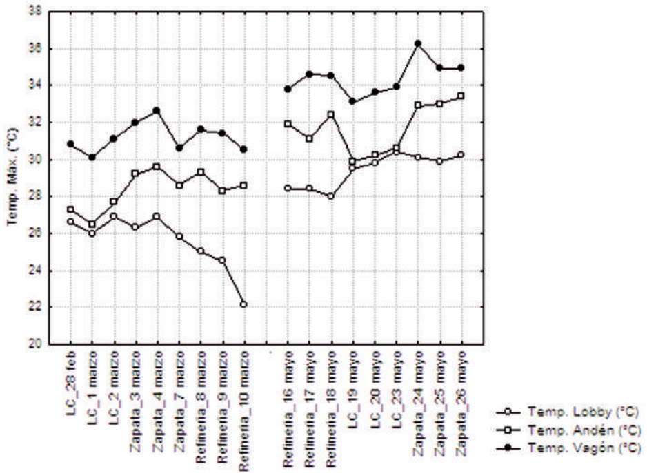
FIG. 3: Temperatura máxima diaria (°C) en lobby, andén y vagón. Campaña fría y cálida.
