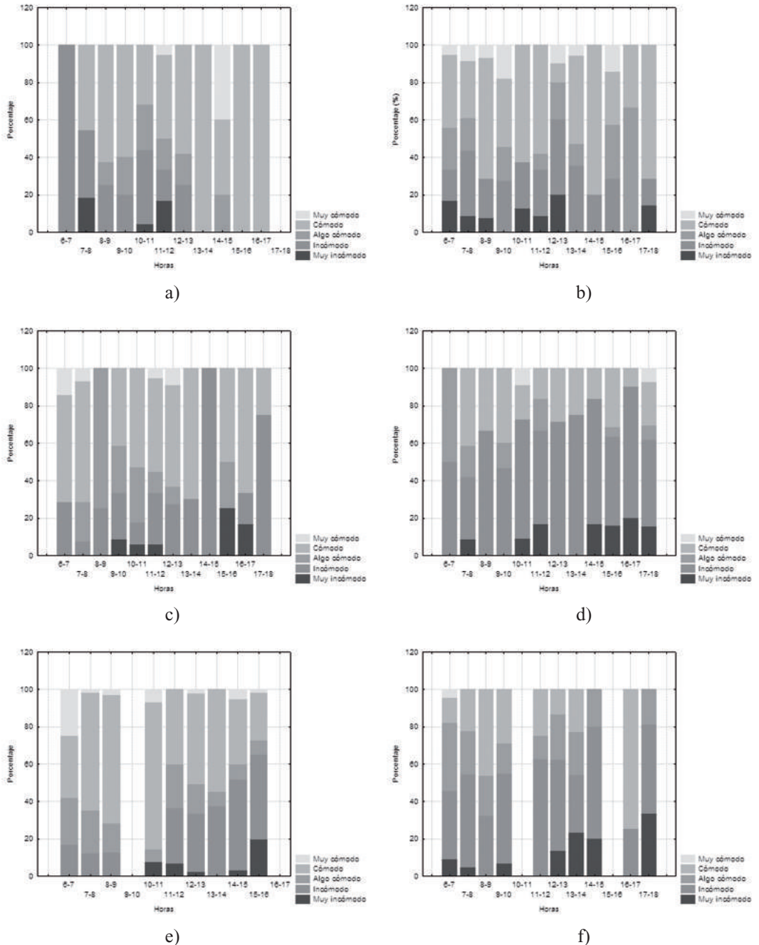
FIG. 5: Comparativo de confort térmico horario en lobby, andén y vagón en época fría a), c) y e) respectivamente; en periodo cálido, b), d) y f) respectivamente.
