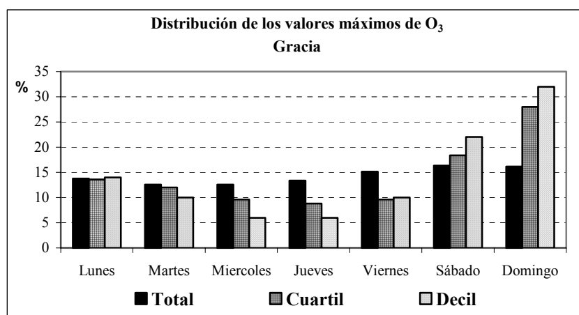
Fig. 10. Distribución, por días de la semana, de las concentraciones de O 3 en Gracia
