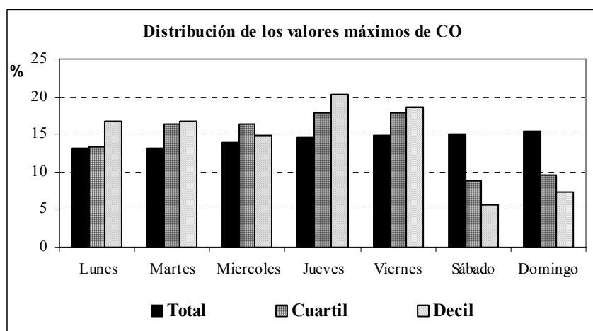
Fig. 2. Distribución, por días de la semana, de las concentraciones de CO
