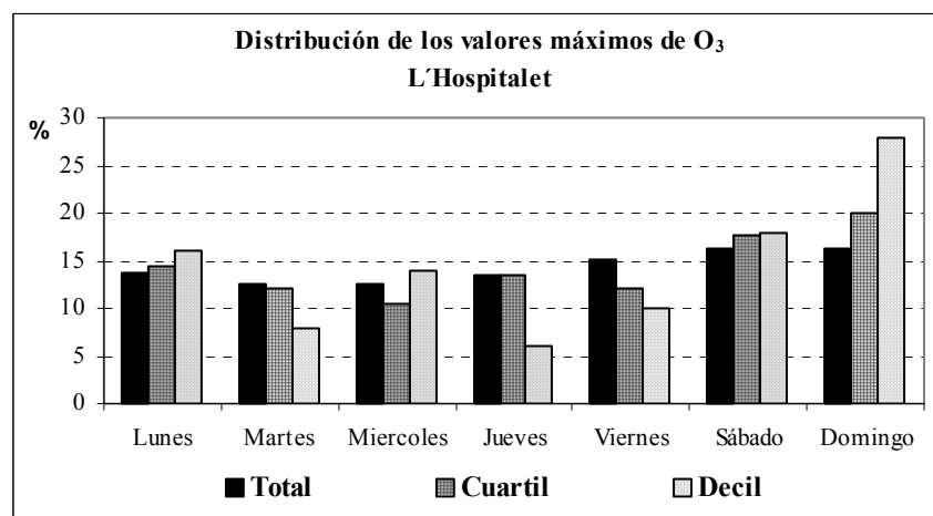
Fig. 9. Distribución, por días de la semana, de las concentraciones de O_3 en L'Hospitalet
