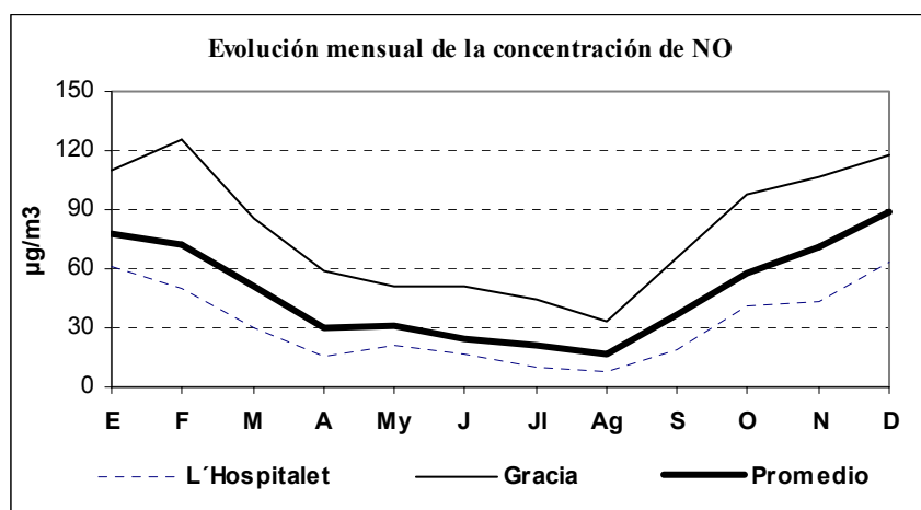
Fig. 8. Evolución de la concentración de NO (Dic. 1998-Nov. 2002)
