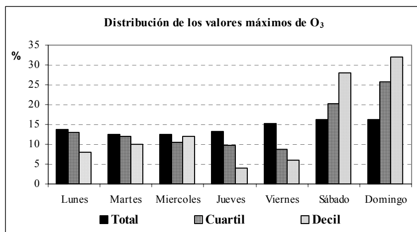
Fig. 6. Distribución, por días de la semana, de las concentraciones de O 3
