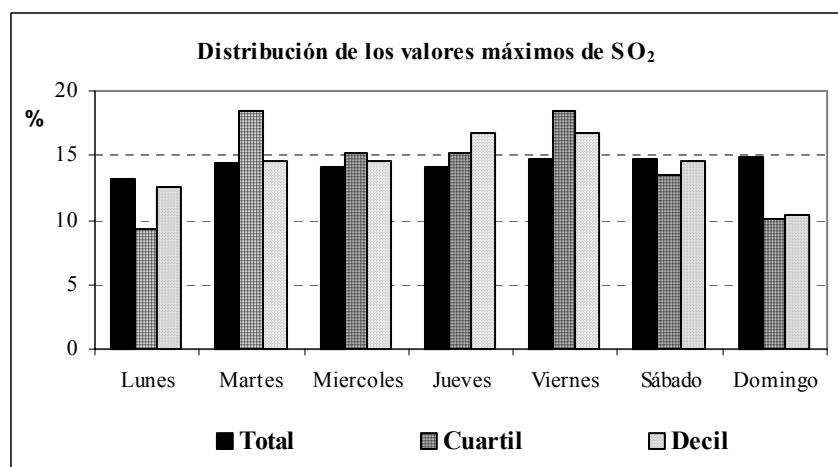
Fig. 3. Distribución, por días de la semana, de las concentraciones de SO 2
