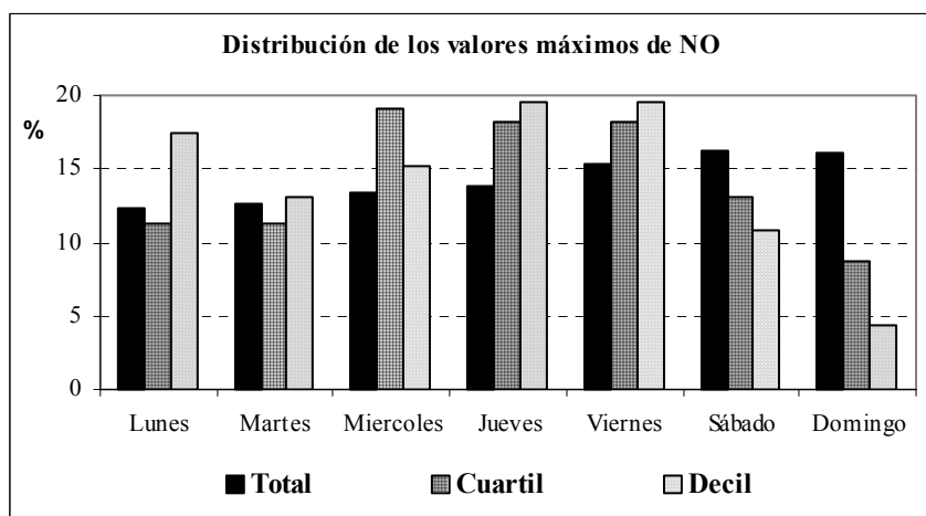
Fig. 4. Distribución, por días de la semana, de las concentraciones de NO
