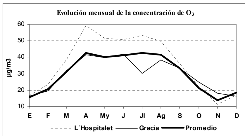
Fig. 7. Evolución de la concentración de O 3 (Dic. 1998-Nov. 2002)
