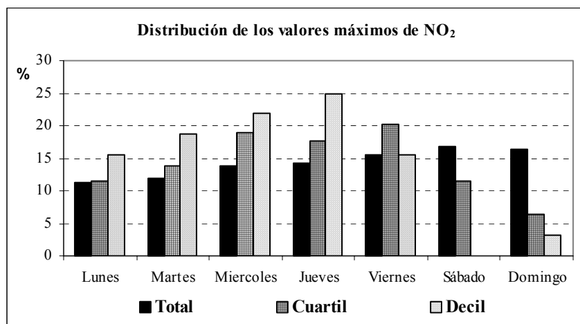
Fig. 5. Distribución, por días de la semana, de las concentraciones de NO 2
