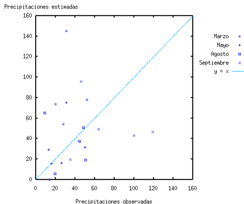
Figura 2. Comparación de las precipitaciones estimadas por 4 ecuaciones de regresión múltiple con las precipitaciones realmente observadas..
