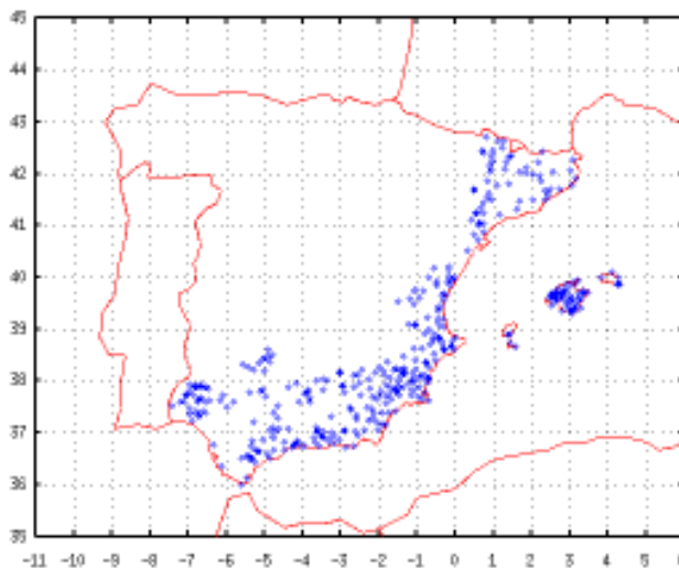
Figura 1. Estaciones pluviométricas de la base de datos utilizada.
