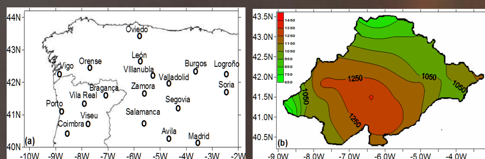
Fig. 1-a: Localización de los observatorios usados en este estudio; b: Distribución de los valores medios anuales de la PET (mm/año), sobre la cuenca del Duero (CD), en el periodo de 1970-2010.
