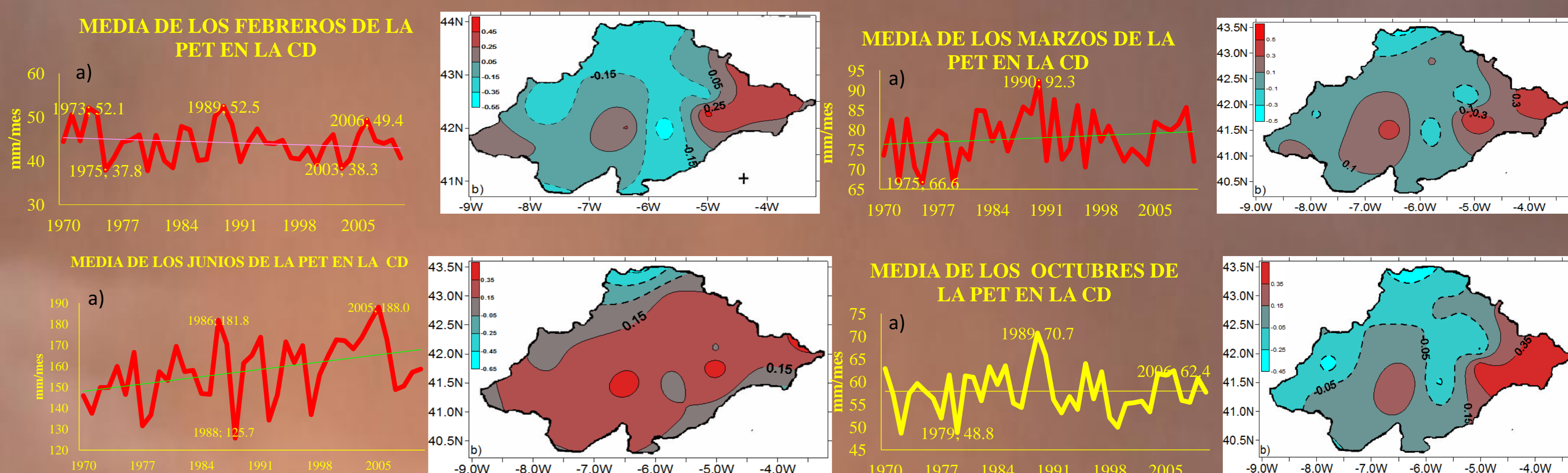
Fig. 2-a: Variación temporal de las medias anual y mensual de la PET en toda la CD; b: Distribución de las tendencias anuales y mensuales de la PET en la CD (mm/año o mm/mes), en el periodo de 1970-2010.
