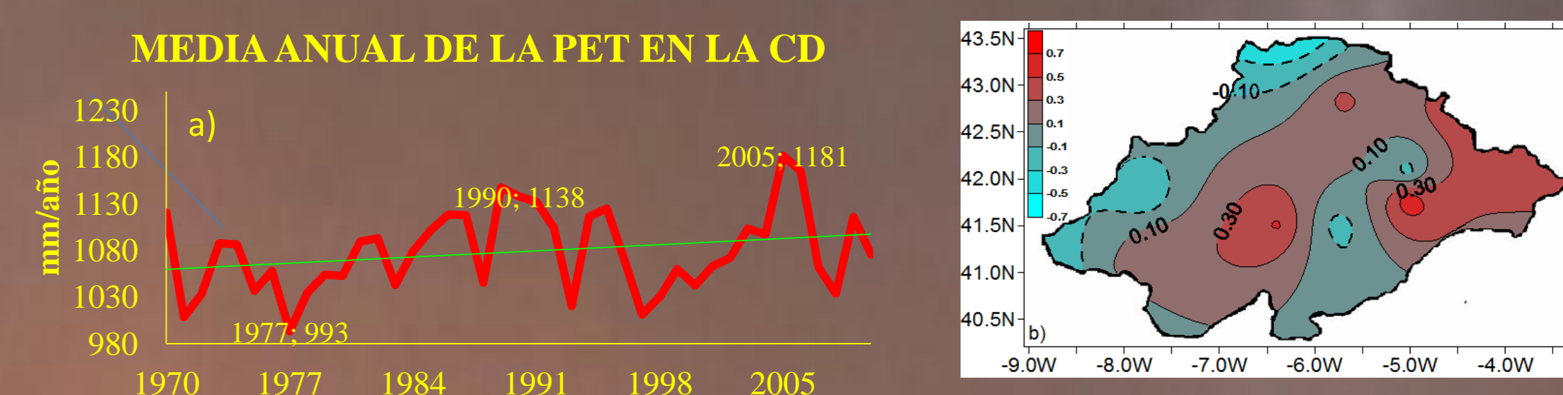
Fig. 2-a: Variación temporal de las medias anual y mensual de la PET en toda la CD; b: Distribución de las tendencias anuales y mensuales de la PET en la CD (mm/año o mm/mes), en el periodo de 1970-2010.
