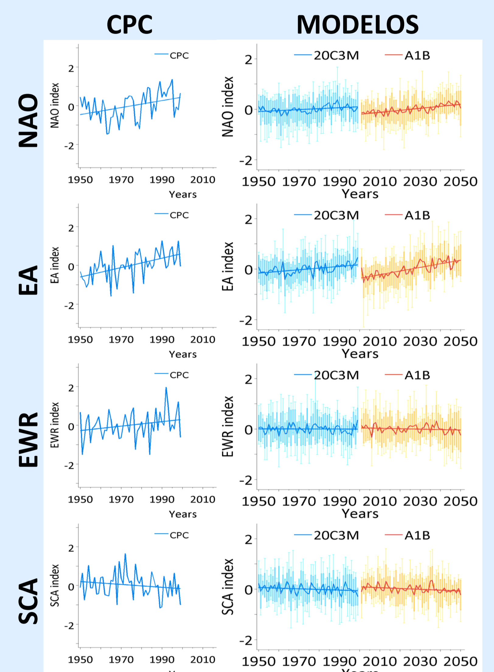
Figura 4: Series temporales de los IT del CPC (primera columna) y del multimodelo (segunda columna). Las líneas gruesas representan la serie temporal y la tendencia, las cajas representan la desviación estándar de entre todos los modelos utilizados en el multimodelo y las barras de error son los valores extremos de los índices.
